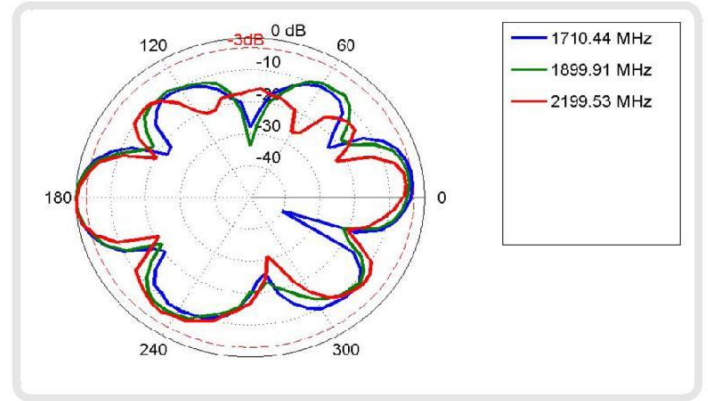
H-Plane: 1700 - 2200 MHz
