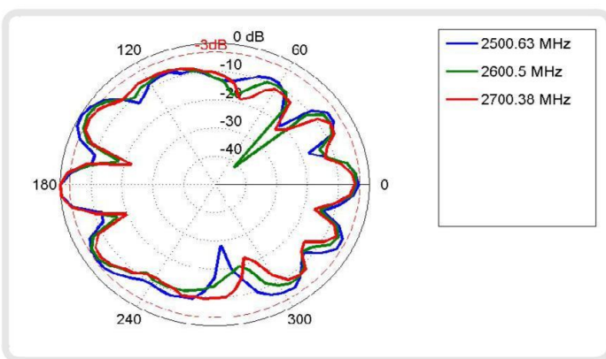
H-Plane: 2500 - 2700 MHz
