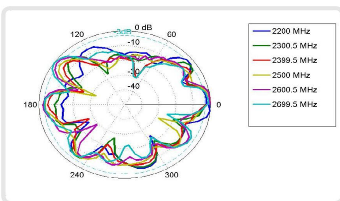
E-Plane: 2200 - 2700 MHz
