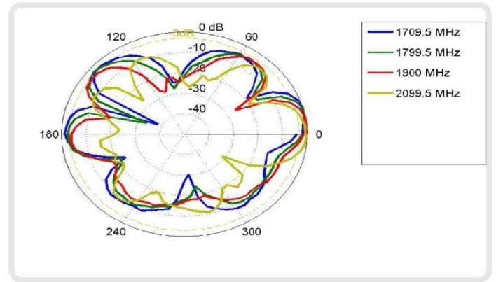
E-Plane: 1700 - 2100 MHz
