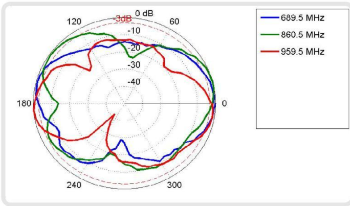
E-Plane: 690 - 960 MHz
